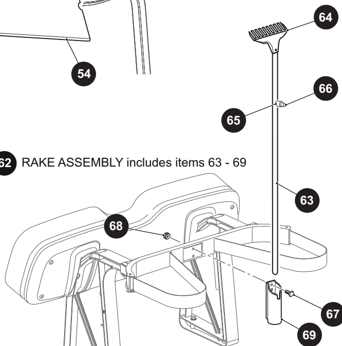
RAKE ASSEMBLY
