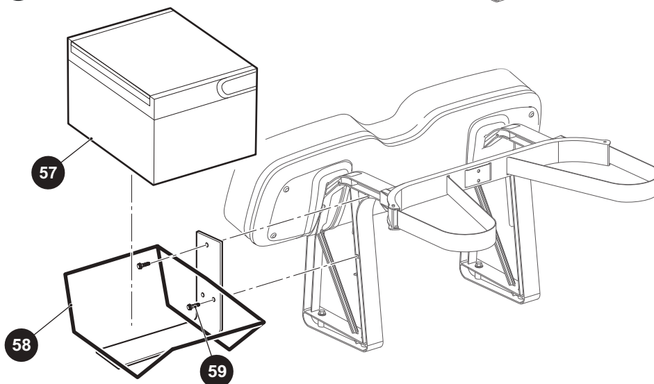
RAKE ASSEMBLY
